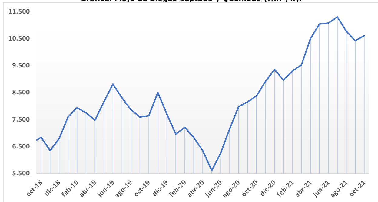
Gráfica. Flujo de Biogás Captado y Quemado (Nm 3 /h).
