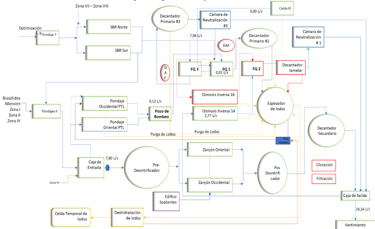
Imagen. Diagrama de flujo octubre 2021
