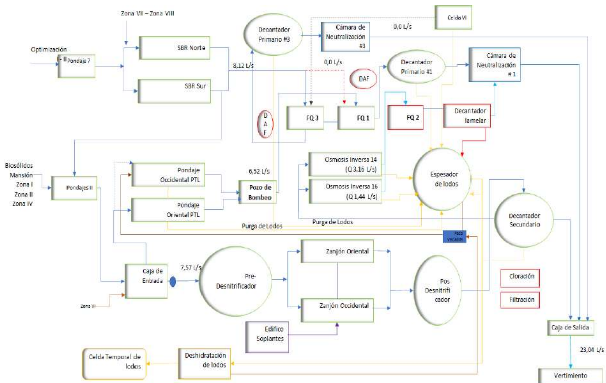
Imagen. Diagrama de flujo abril 2021
