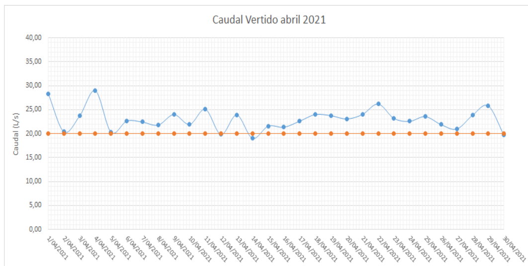
Gráfica. Comportamiento caudal vertido FT -11 – abril 2021
