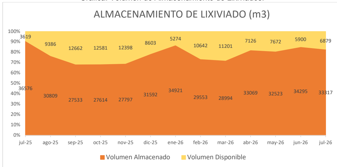
Gráfica. Volumen de Almacenamiento de Lixiviados.
