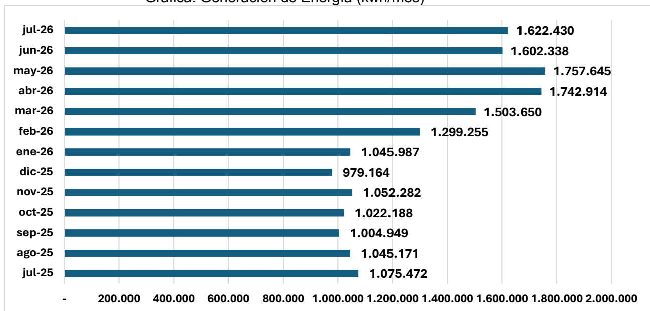
Grafica. Generación de Energía (kwh/mes)
