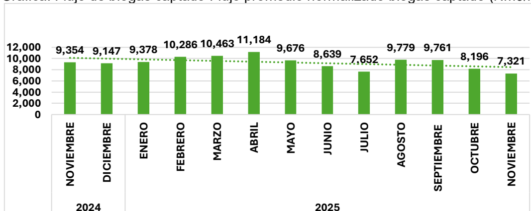
Grafica. Flujo de biogás captado Flujo promedio normalizado biogás captado (Nm3/h)
