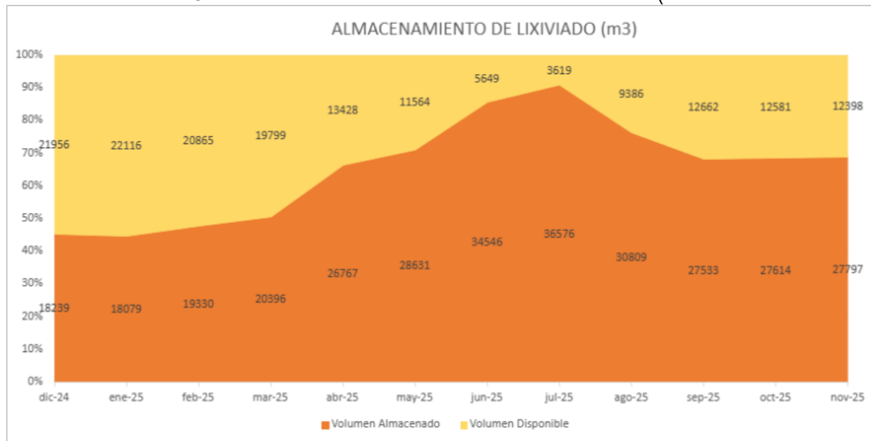
Gráfica. Volumen de Almacenamiento de Lixiviados.( m 3 )
