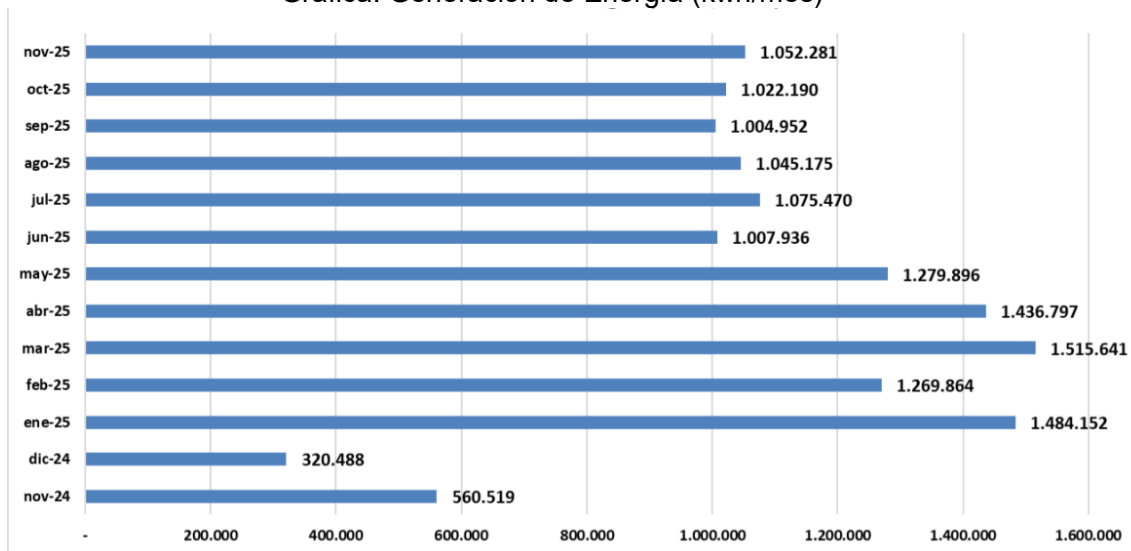
Grafica. Generación de Energía (kwh/mes)
