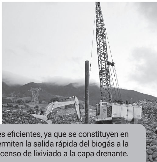
» 3. Chimeneas perforadas (verticales), las cuales mediante la introducción de una bomba se extrae el lixiviado presente en las zonas de altas presiones.
